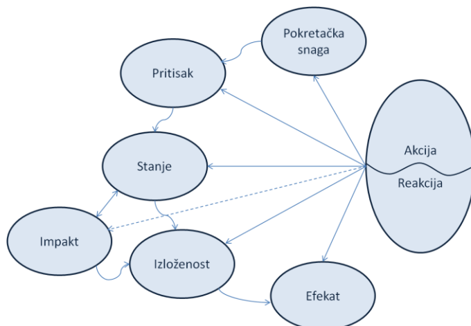
Slika 3.DPSIEERA metodologija
